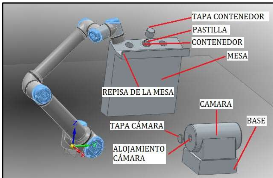
Fig. 1 – Modelo 3D de la celda de trabajo
