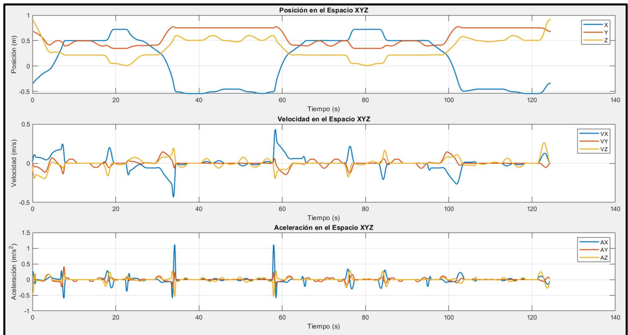
Fig. 32 – Gráficos de posición, velocidad y aceleración en el espacio cartesiano.
