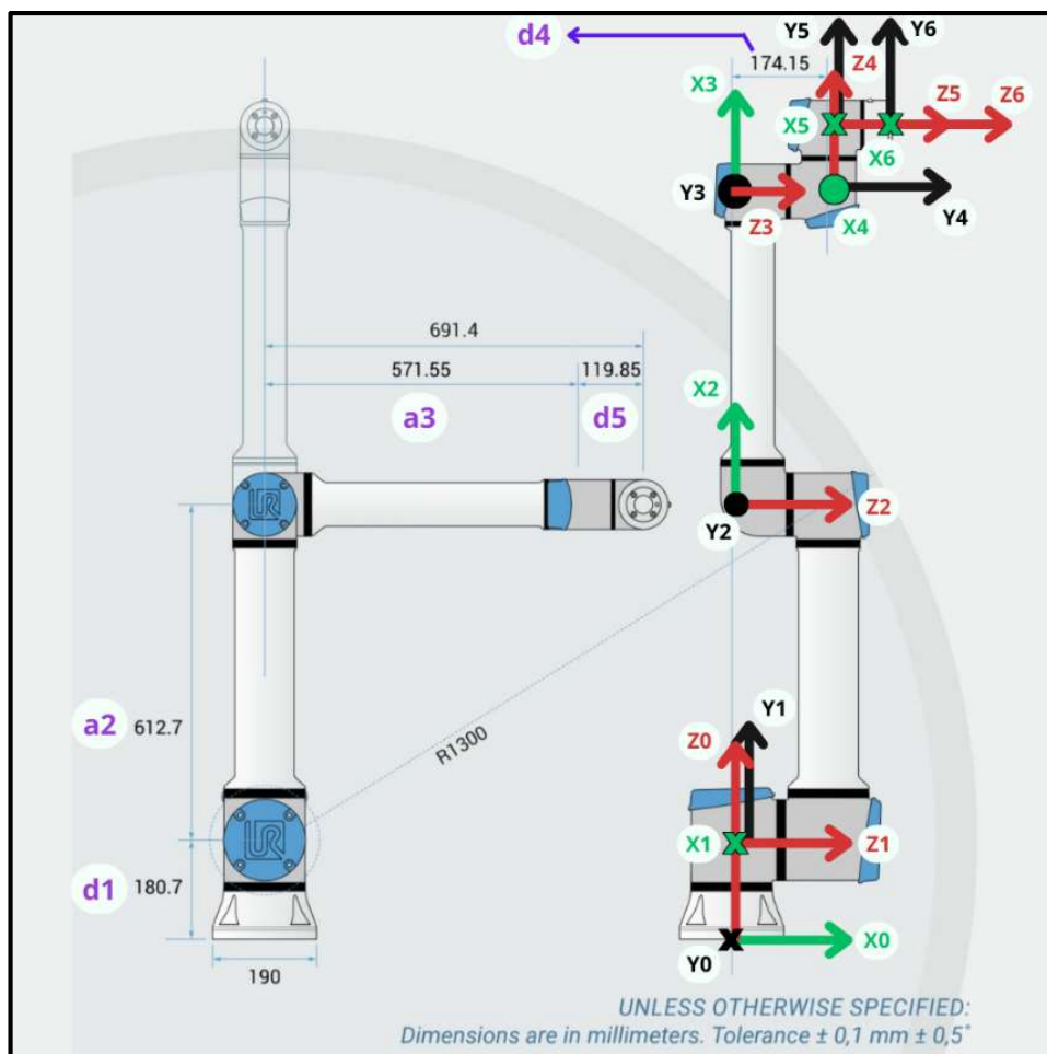
Fig. 13 – Aplicación de la convención de Denavit-Hartenberg
