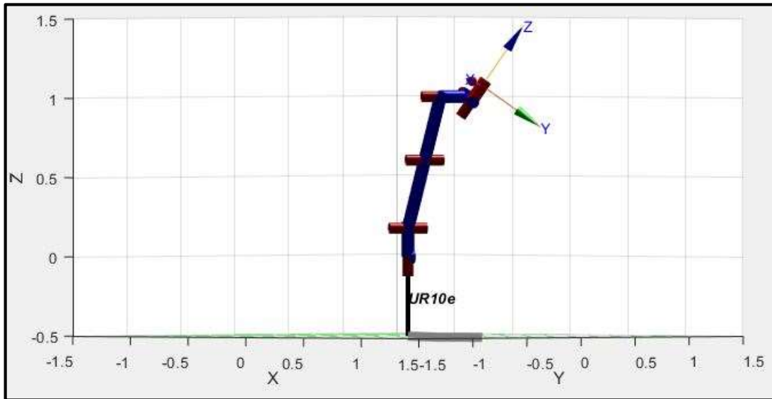
Fig. 16 – Ejemplo Singularidad de codo.
