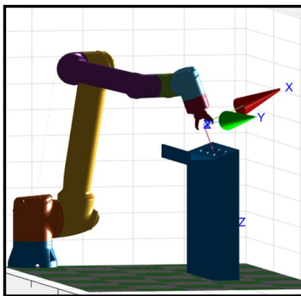
Fig. 24 – Enfrentamiento al contenedor
