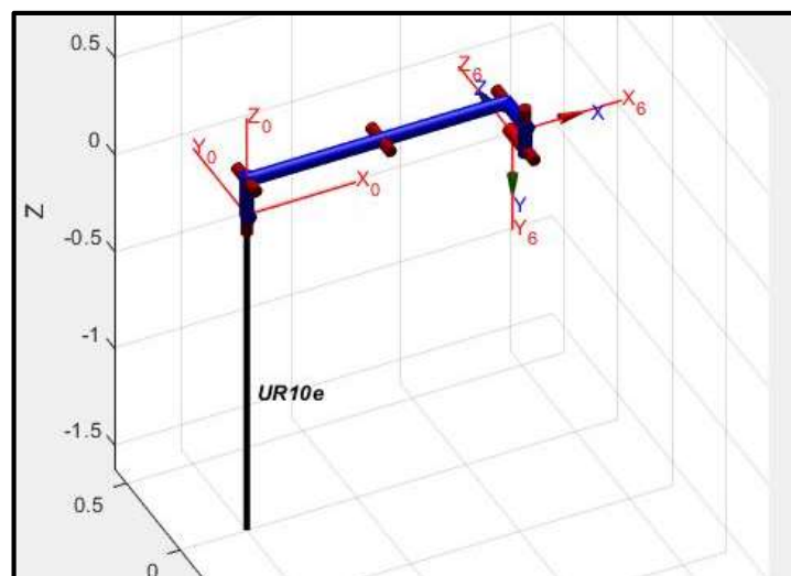
Fig. 14 – Posición zero con offset nulo
